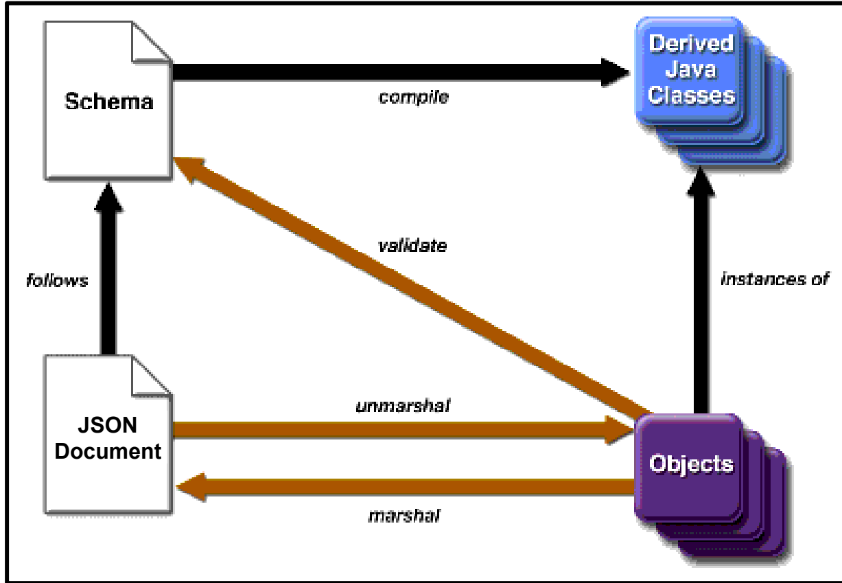
JSON-OOP data binding
